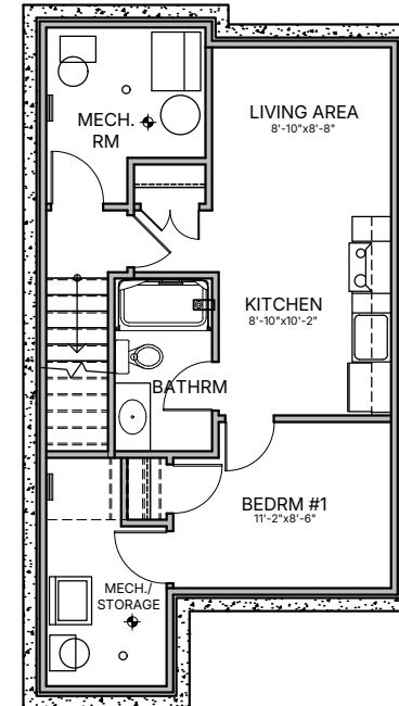
OPTIONAL BASEMENT SUITE LAYOUT - 653 sq.ft.
