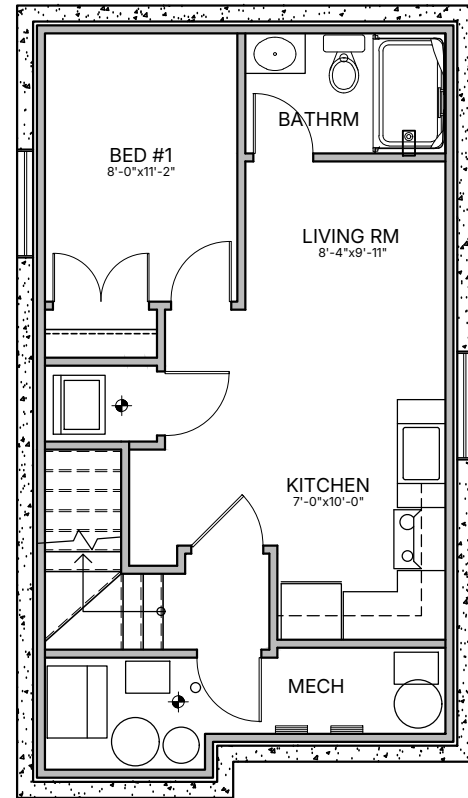
OPTIONAL BASEMENT SUITE LAYOUT - 612 sq.ft.
